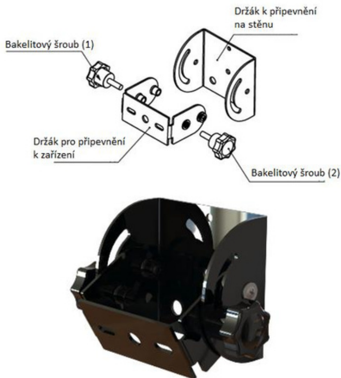
Schéma 2 Montáž aparátu
