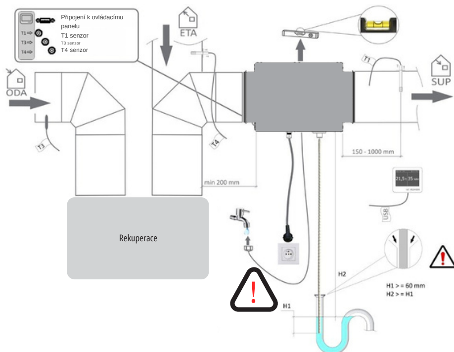
Obr. 4. Schéma instalace zvlhčovače HUMON
